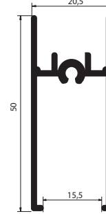
SR 1775 NEW! 8-18 mm Alt Kayıt
