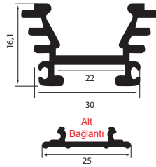
ÇP 0008 A NEW! Alüminyum Led Profili
