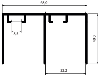
Çift Frenli Üst Ray
