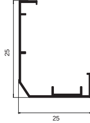
ÇP 0007 B NEW! Alüminyum Led Profili
