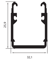
ÇP 0005 B NEW! Alüminyum Led Profili
