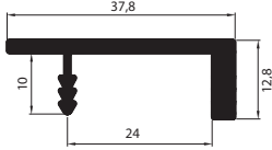
MD 1033 18 S Chipboard F Kulp
