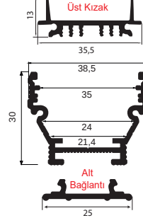
ÇP 0007 C NEW! Alüminyum Led Profili
