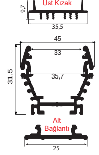
ÇP 0007 D NEW! Alüminyum Led Profili
