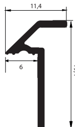
MD 1027 T NEW! Cam Çıtası / Glass Molding
