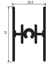
SR 1778 NEW! 8-18 mm Ara Kayıt
