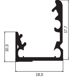
ÇP 0002 C NEW! Alüminyum Led Profili
