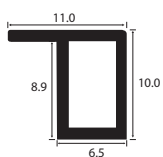
MD 1093 A NEW! Cam Çıtası / Glass Molding
