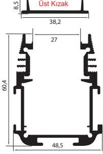
ÇP 0008 NEW! Alüminyum Led Profili
