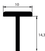
MD 1027 S NEW! Cam Çıtası / Glass Molding
