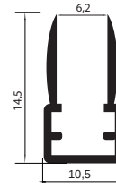
ÇP 0008 C NEW! Alüminyum Led Profili
