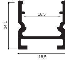
ÇP 0003 B NEW! Alüminyum Led Profili
