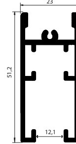
SR 2738 NEW! 8-18 mm Alt Kayıt
